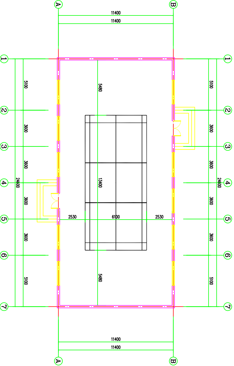
羽毛球场地划线平面图 蓝色油漆
