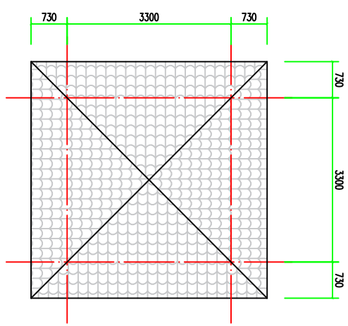
木亭梁平面示意图
