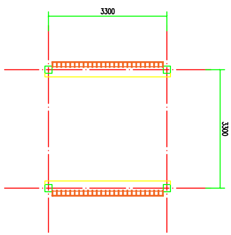
木亭梁平面示意图
