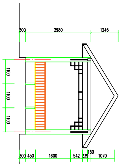
木亭东立面示意图
