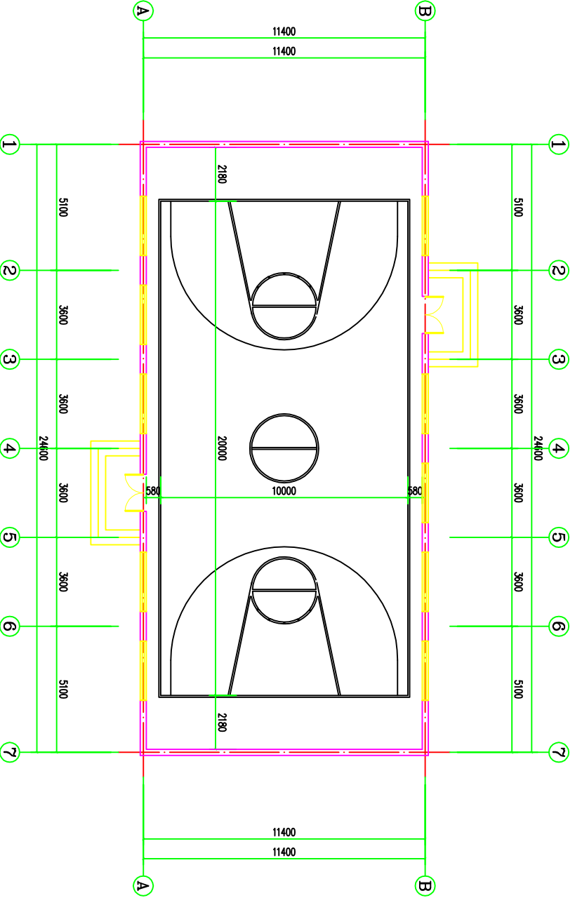
篮球场划线平面图 白色油漆
