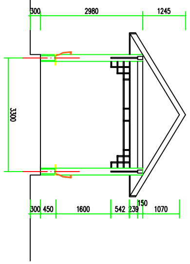
木亭南立面示意图
