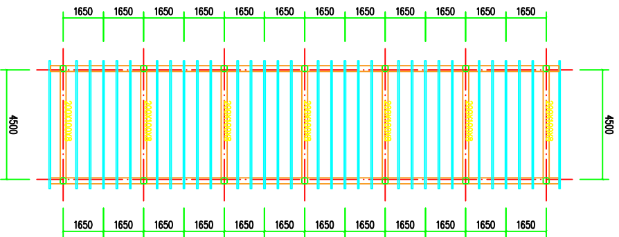
改造后梁及标条平面图
