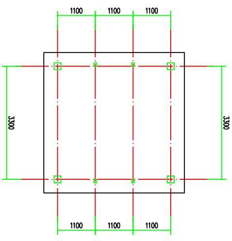
木亭柱平面示意图
